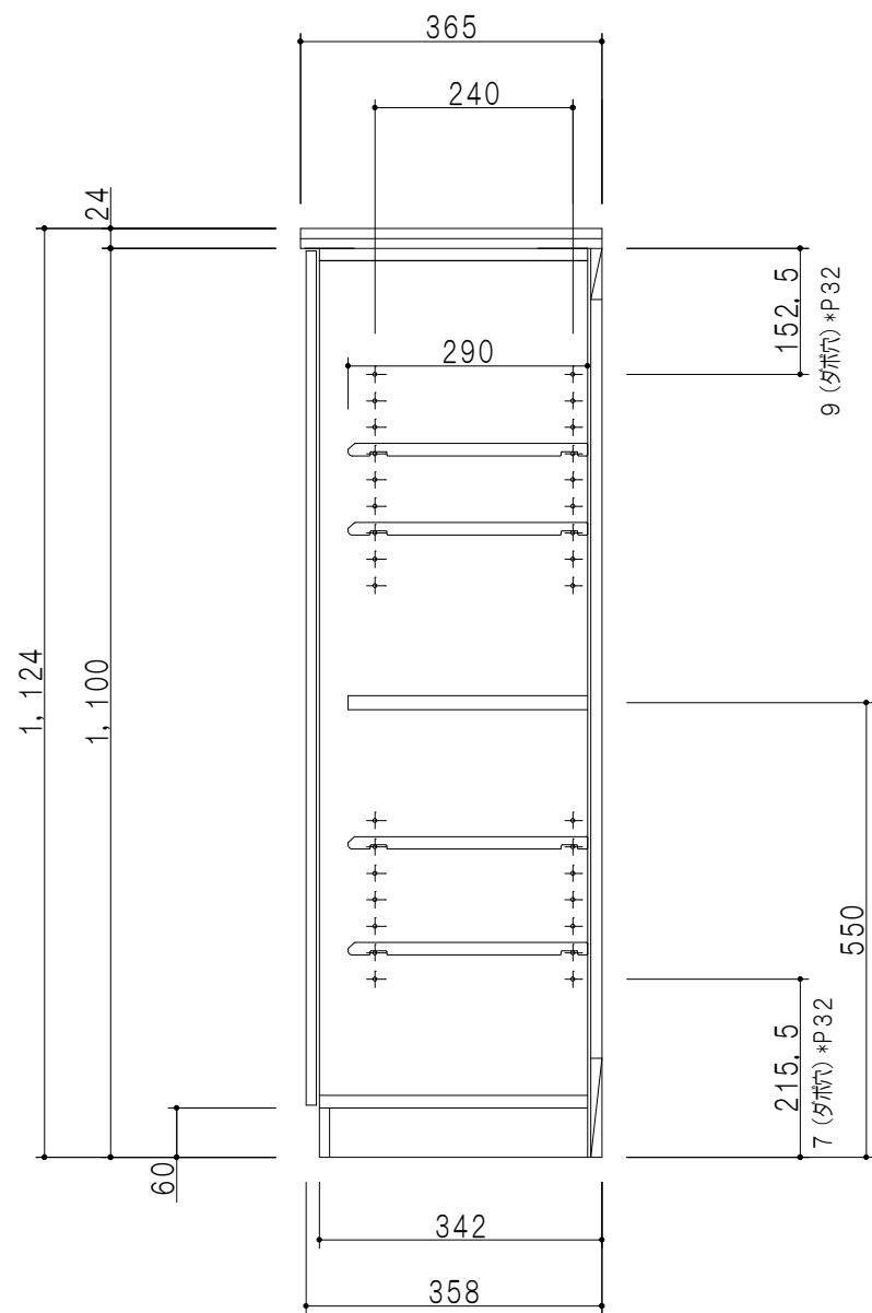
断面図
