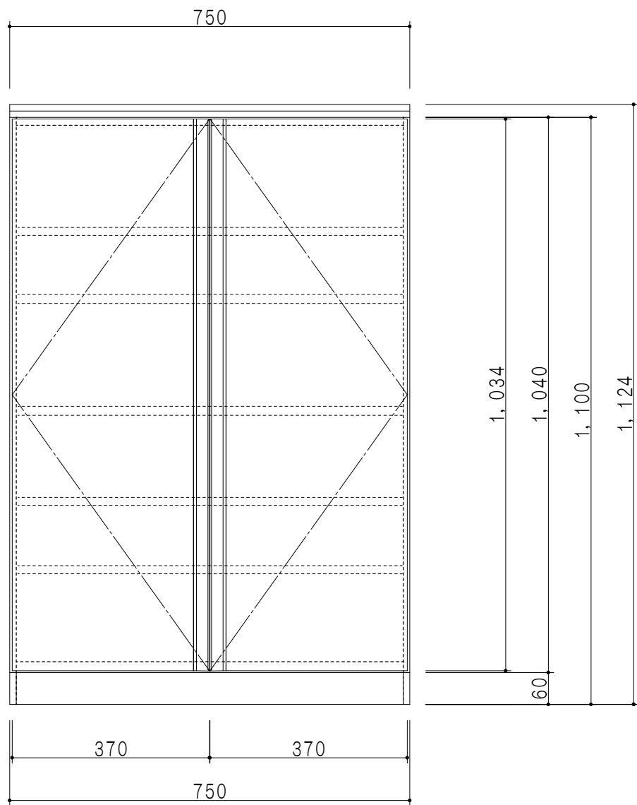
立面図
