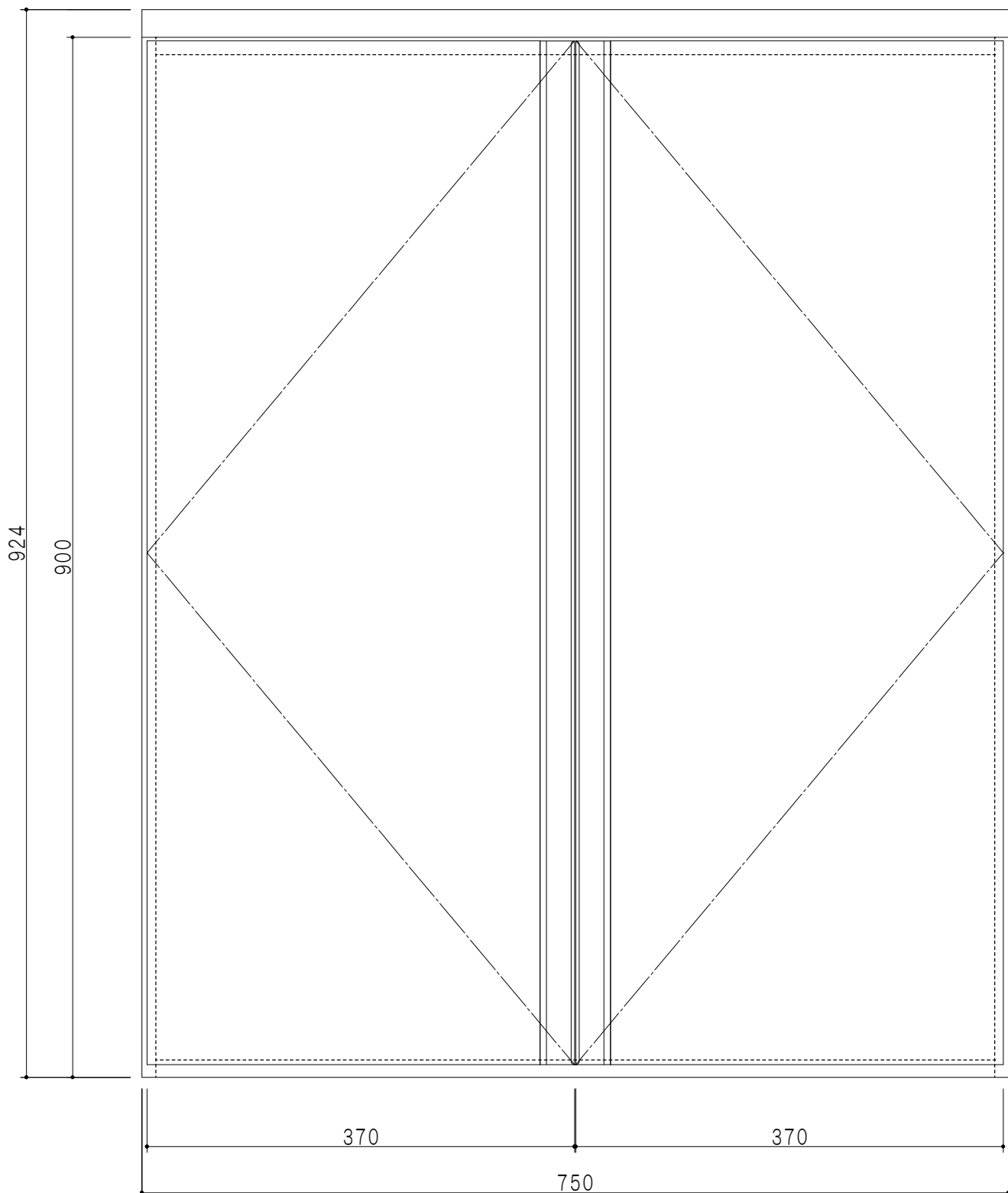
立面図
