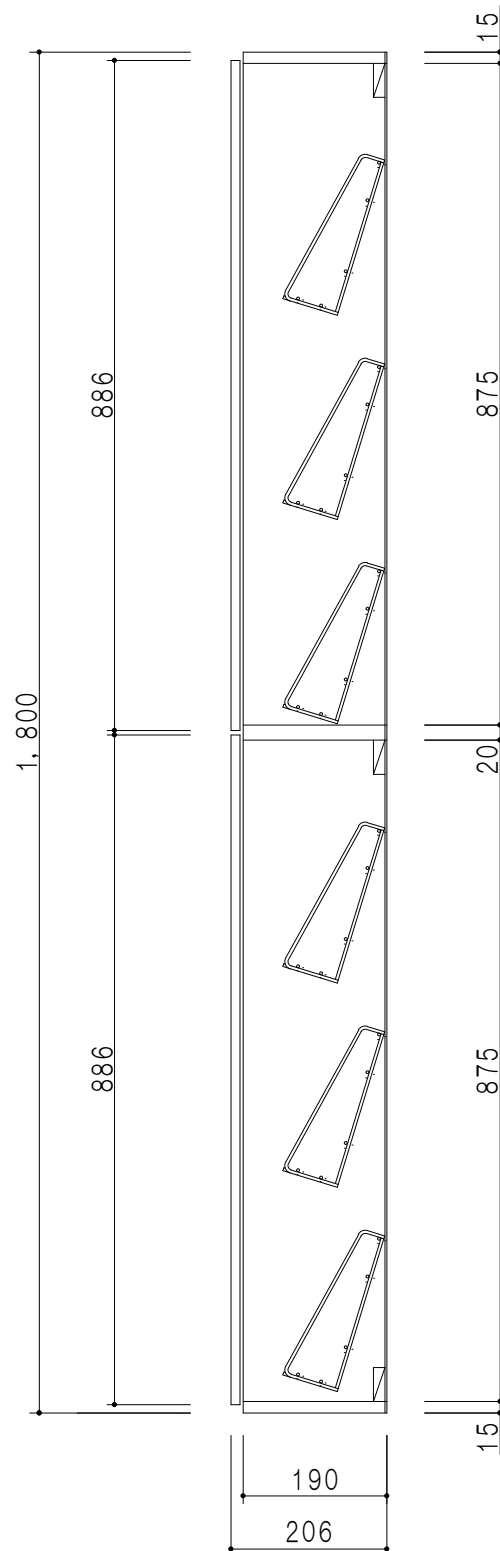
断面図
