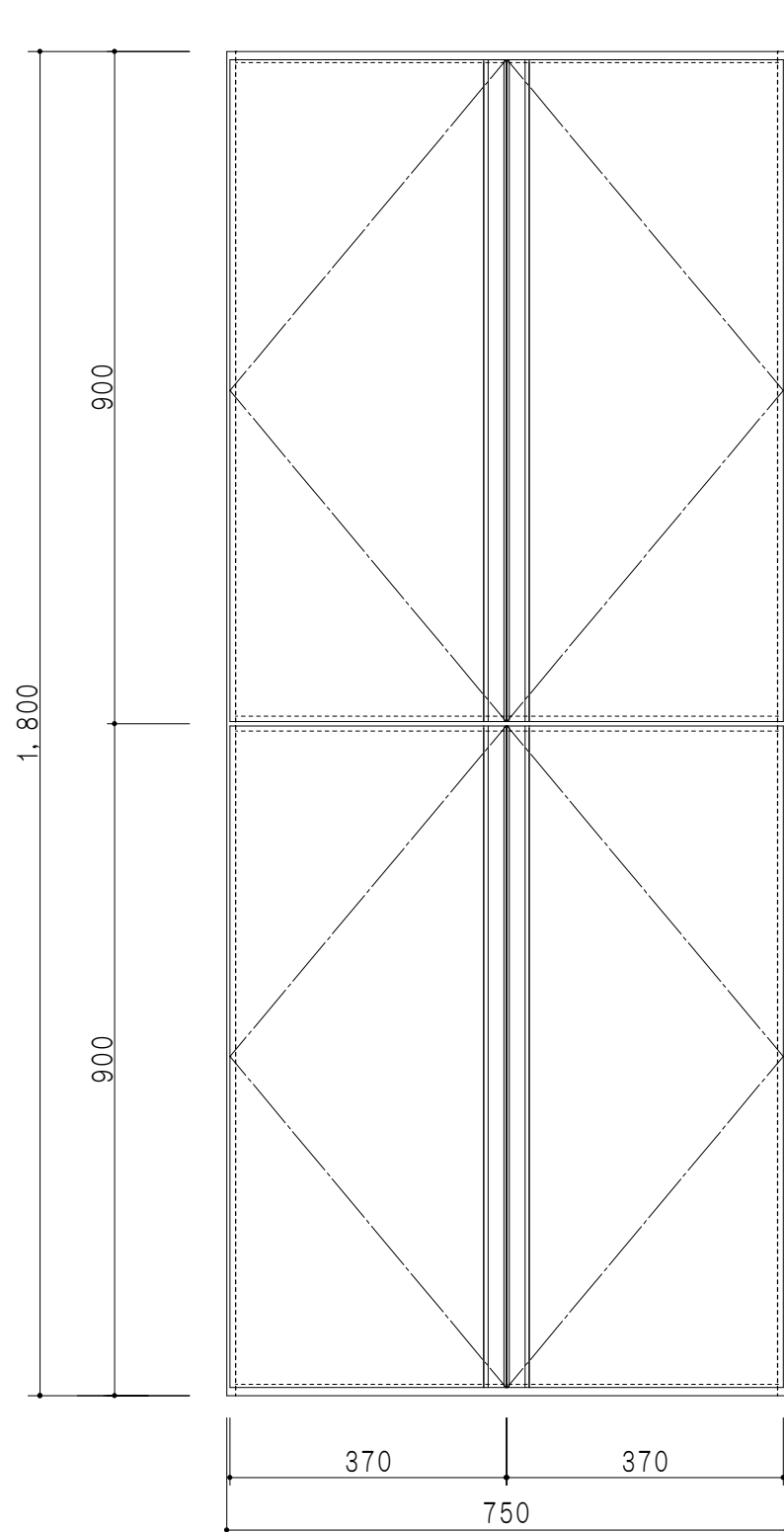
立面図
