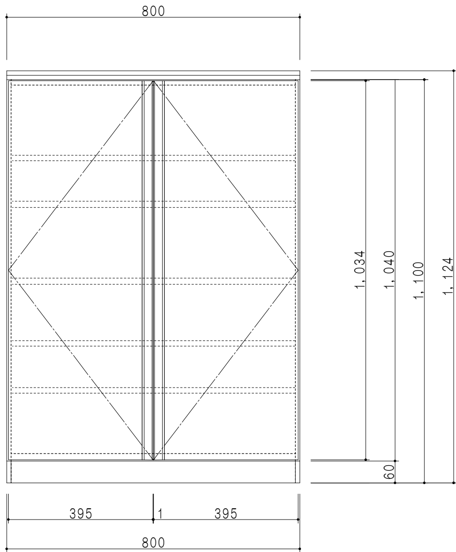
立面図
