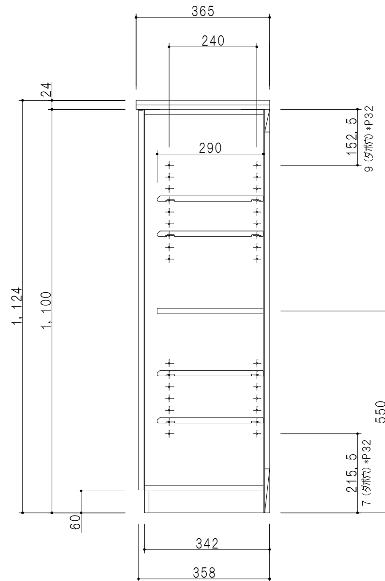
断面図
