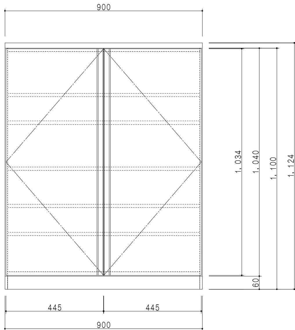
立面図
