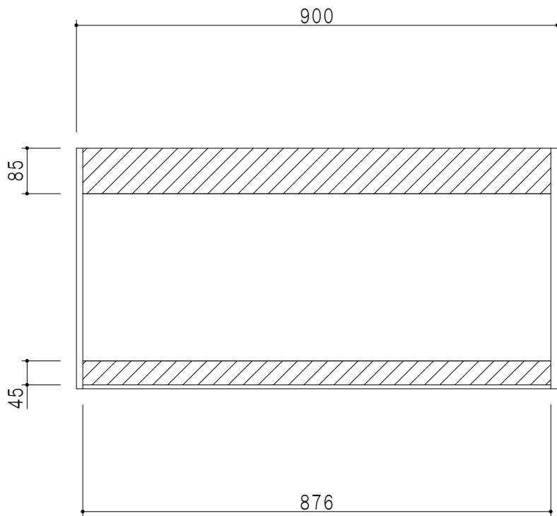
背面図
