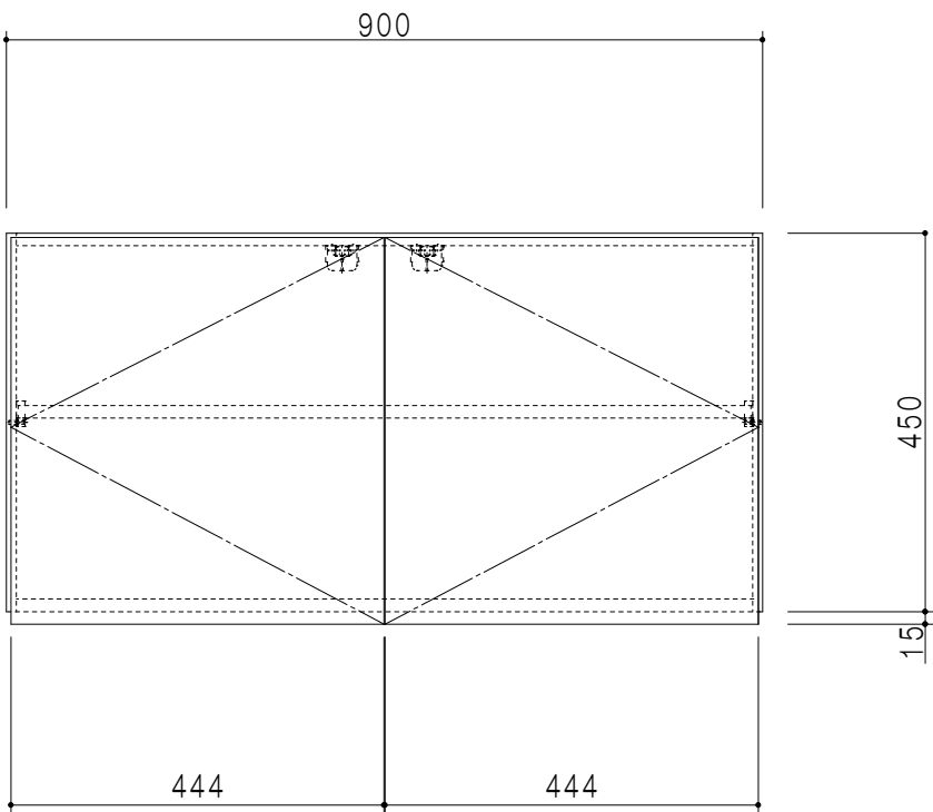
立面図
