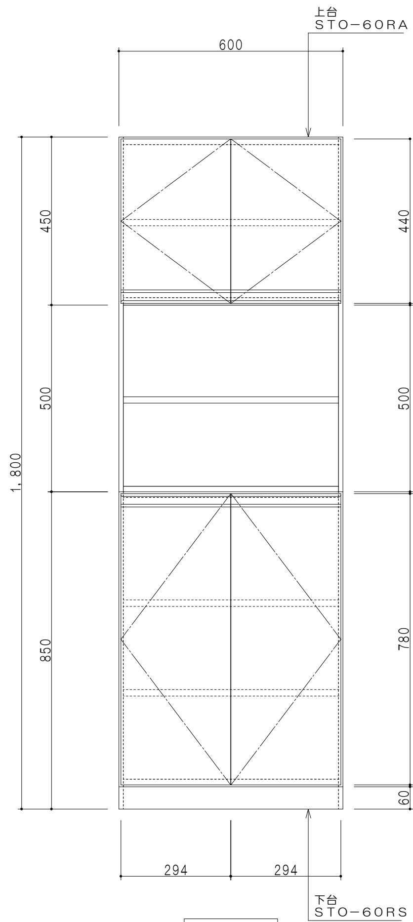
立面图
