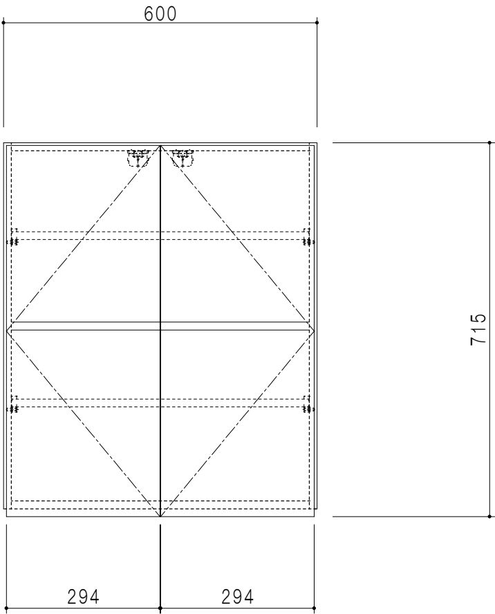
立面図
