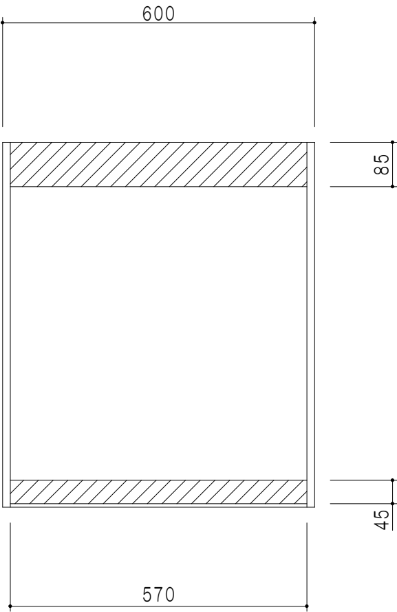
背面図
