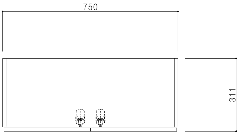
平面図
