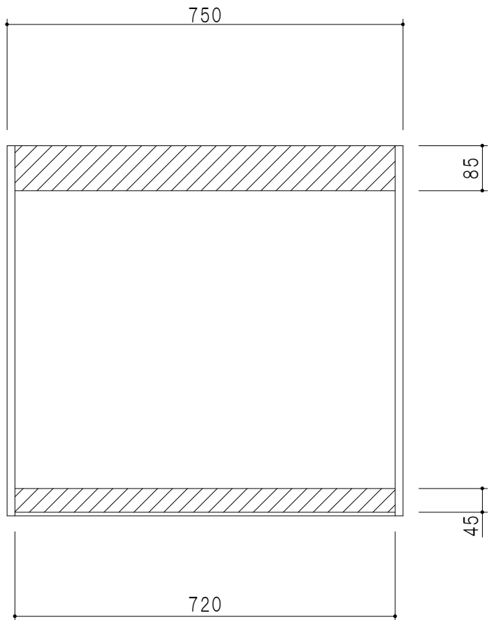
背面図
