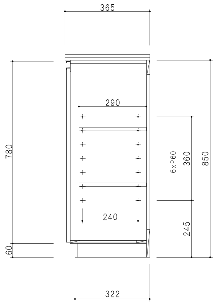
断面図
