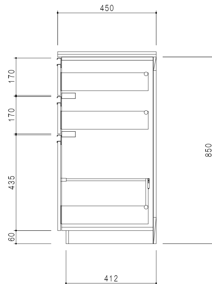
断面図
