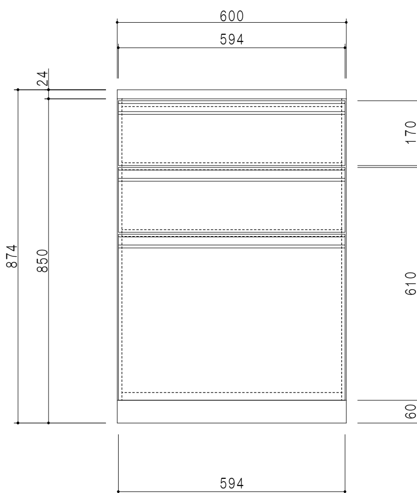
立面図
