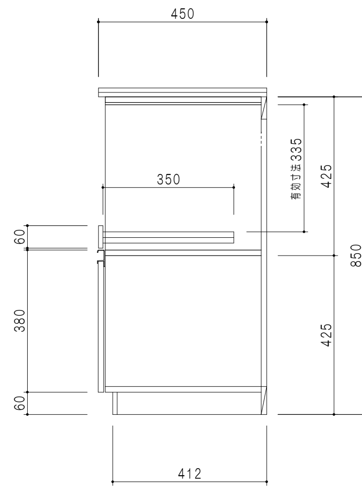
断面図
