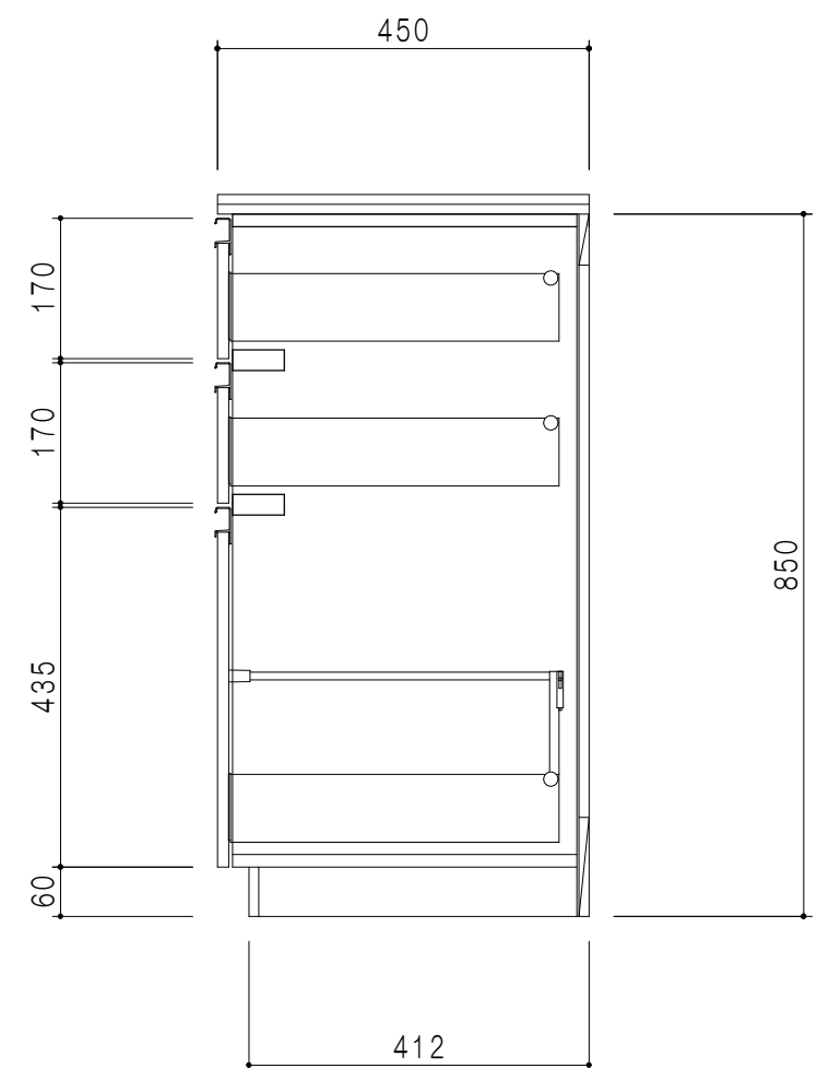
断面図
