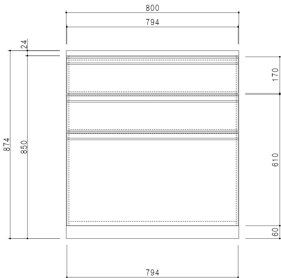
立面図
