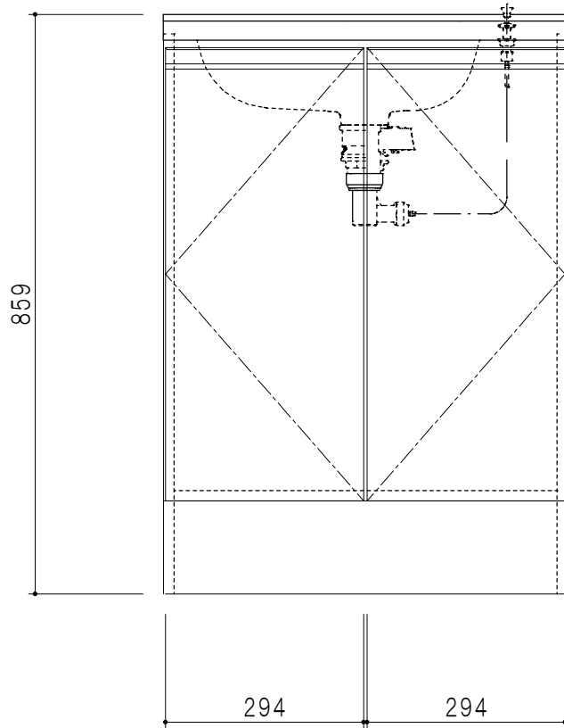
立面図
