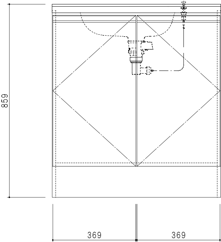
立面図
