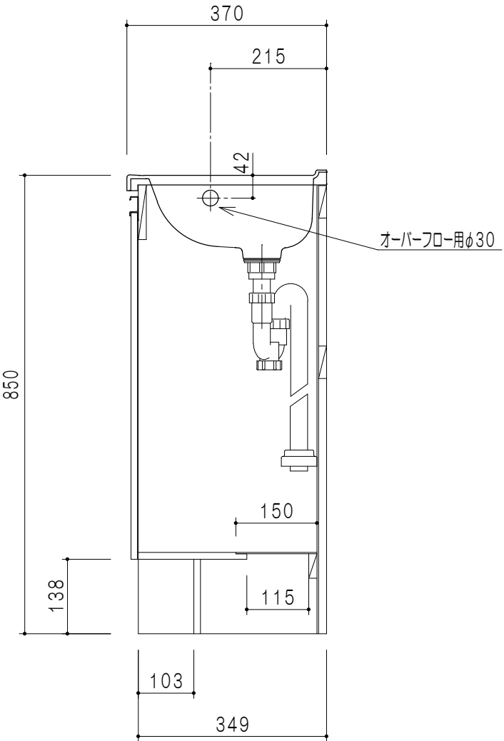
断面図
