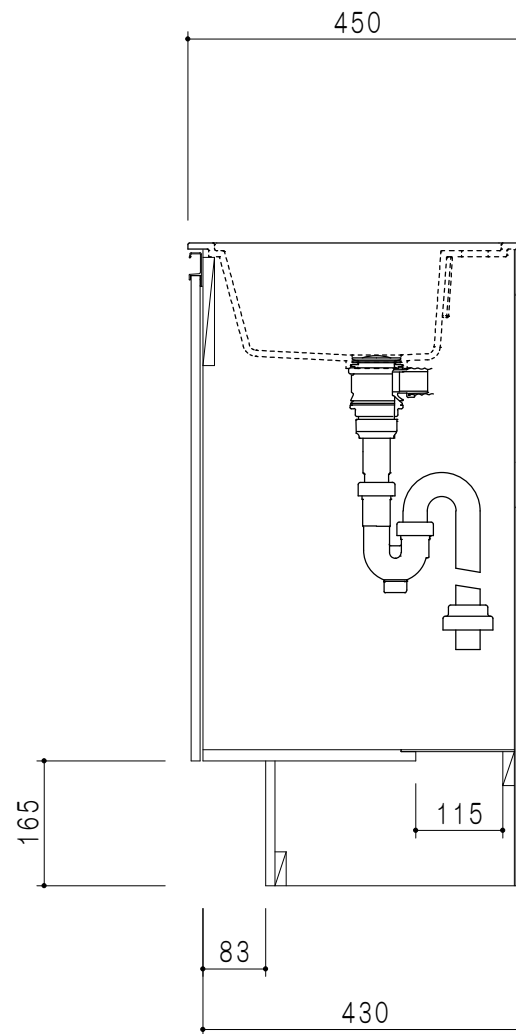
断面図
