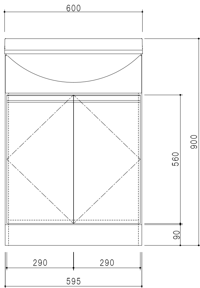
立面図
