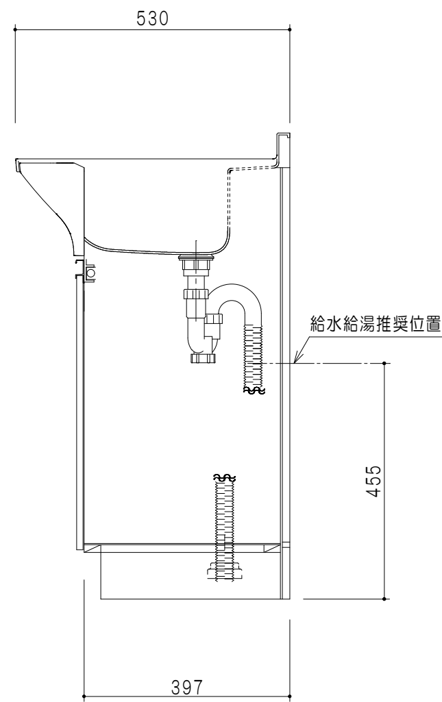
断面図
