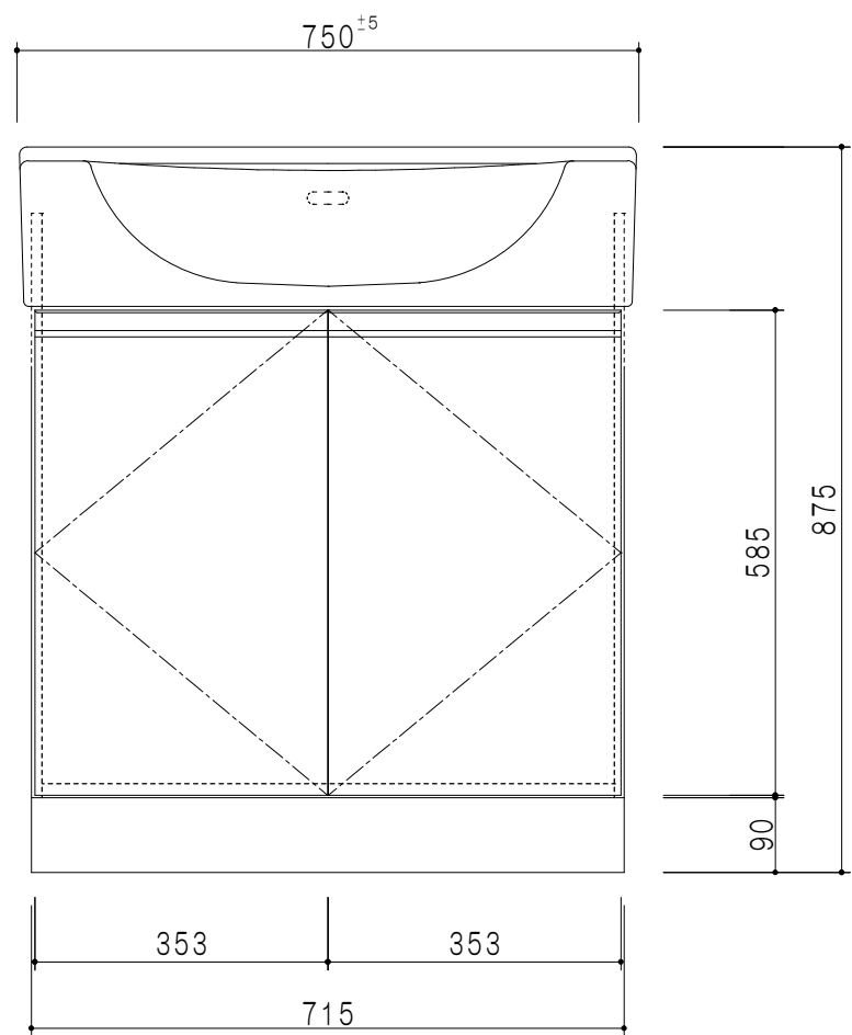
立面図
