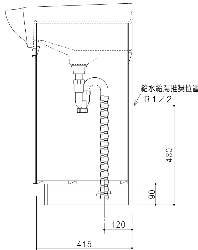
断面図
