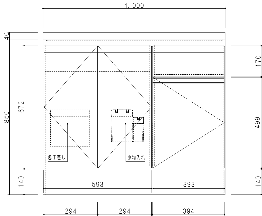
立面図
