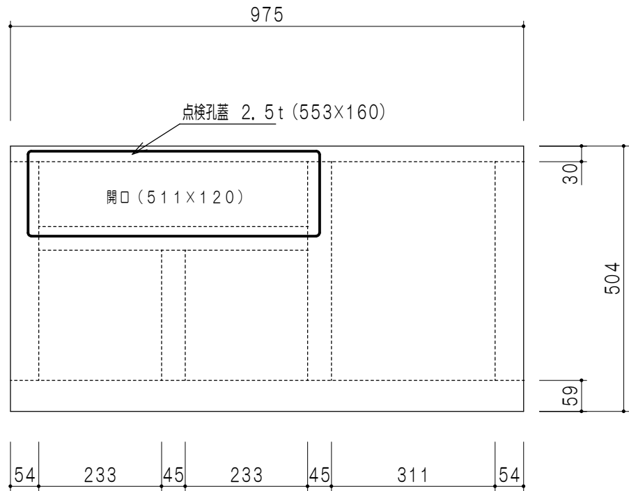
地板詳細
