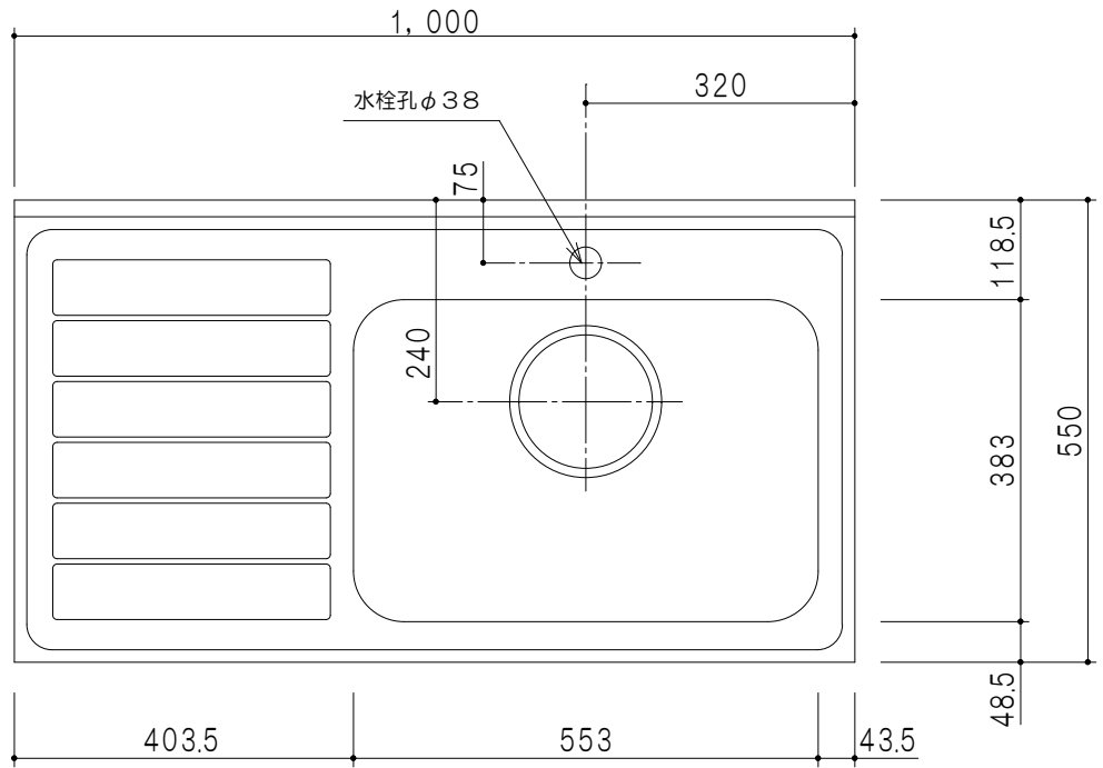
平面図
