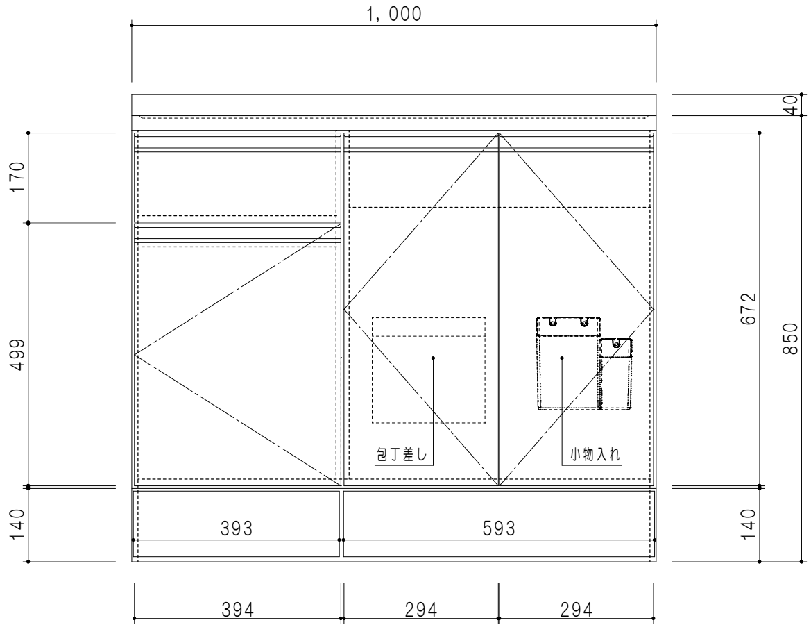
立面図
