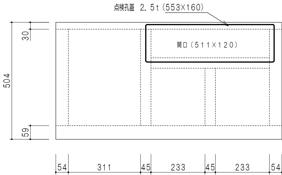
地板詳細
