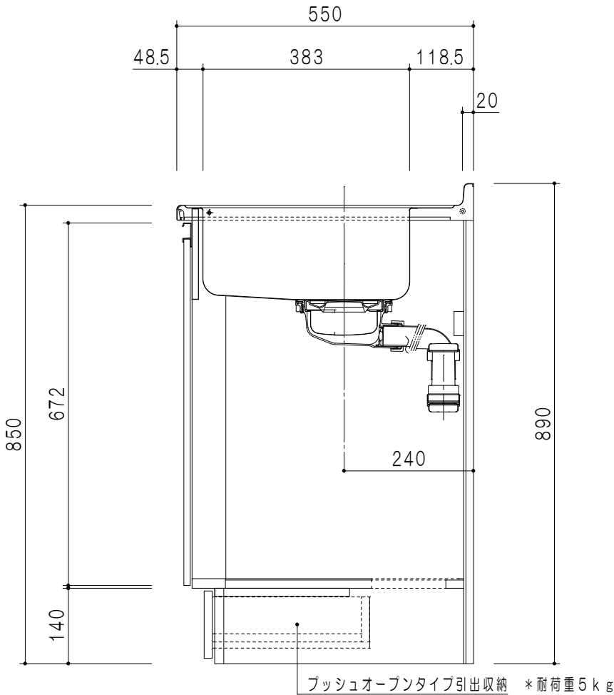
地板詳細
