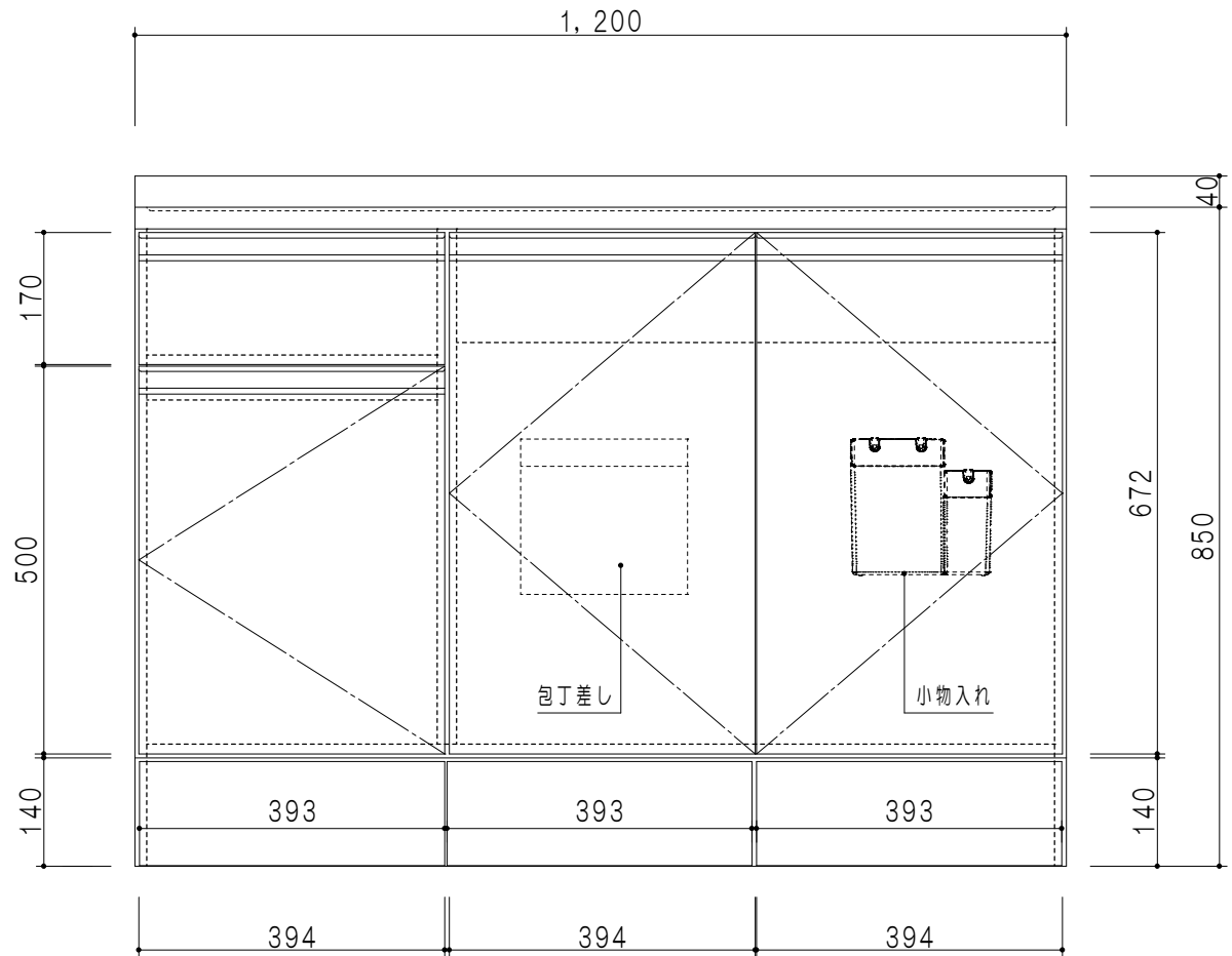
立面図
