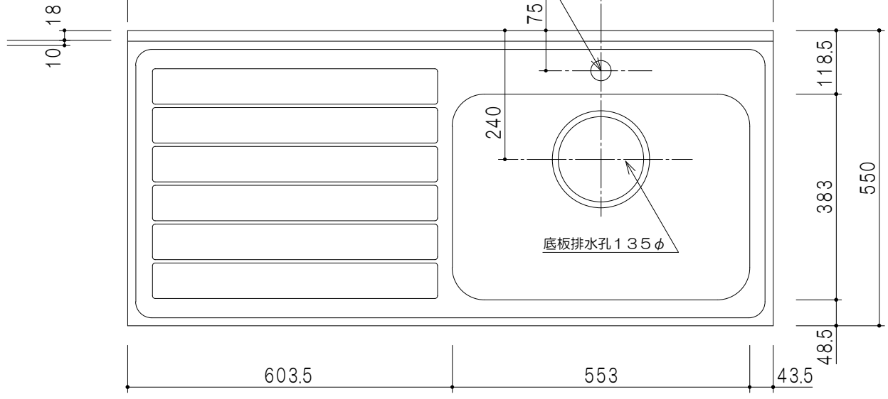
平面図
