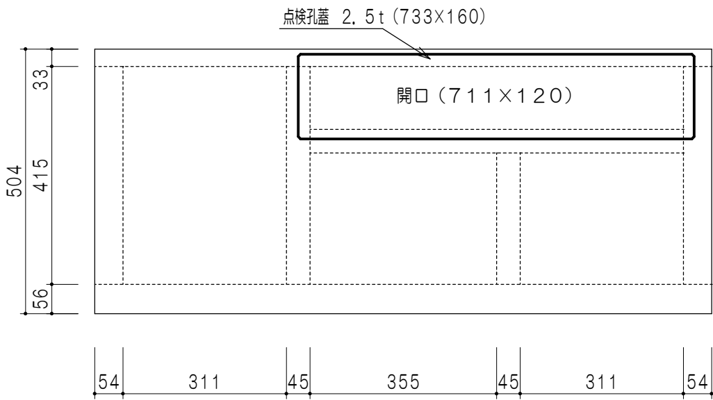
地板詳細
