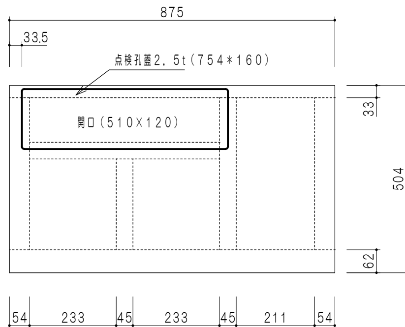
地板詳細
