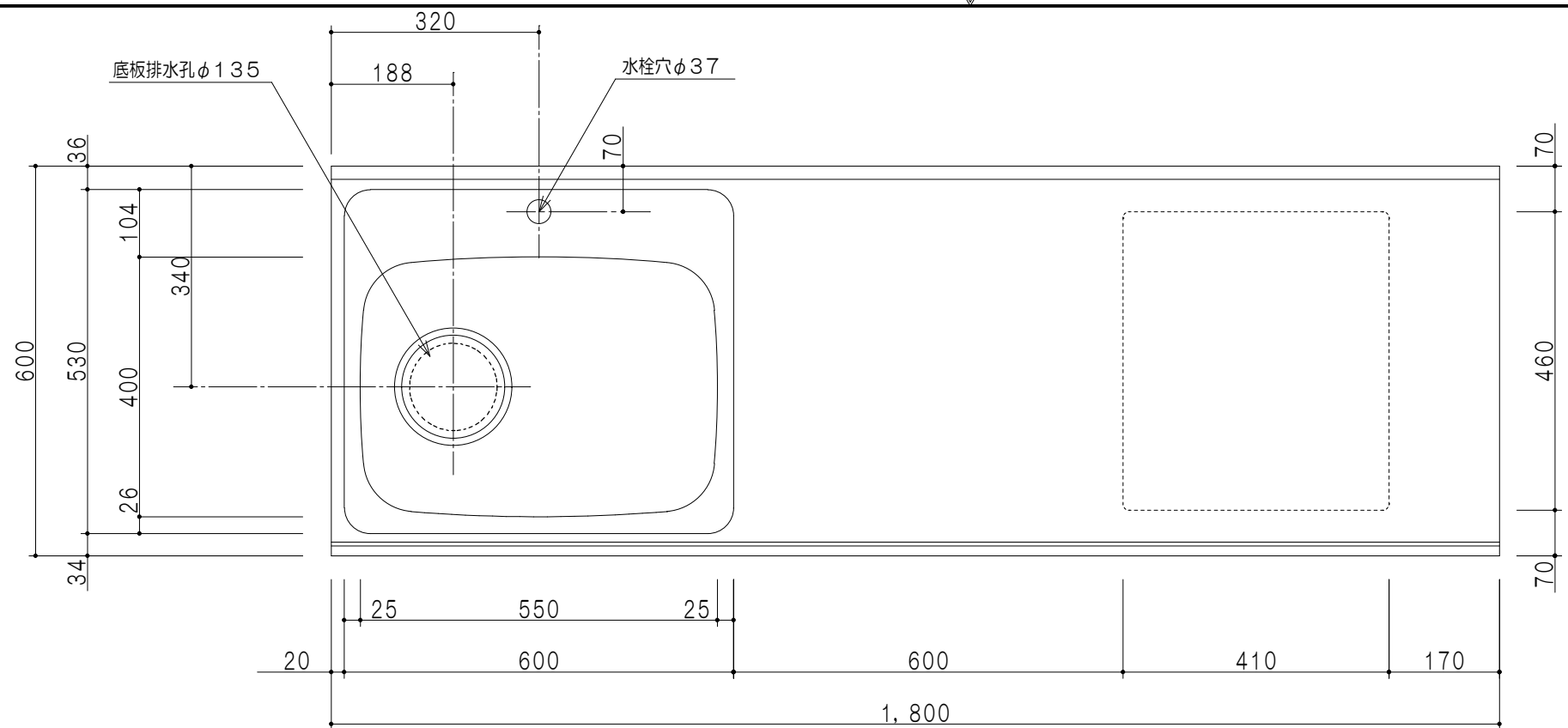
平面図
