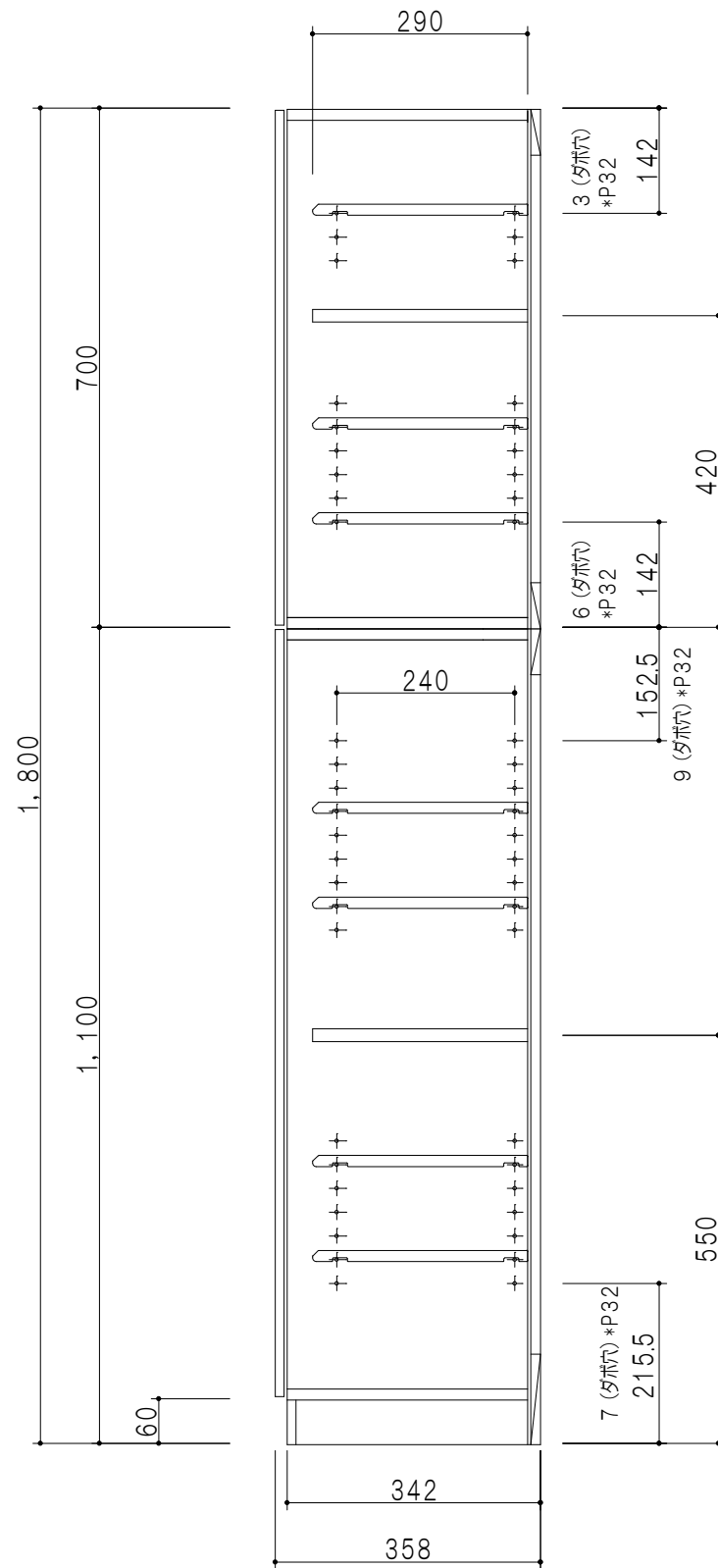
断面図
