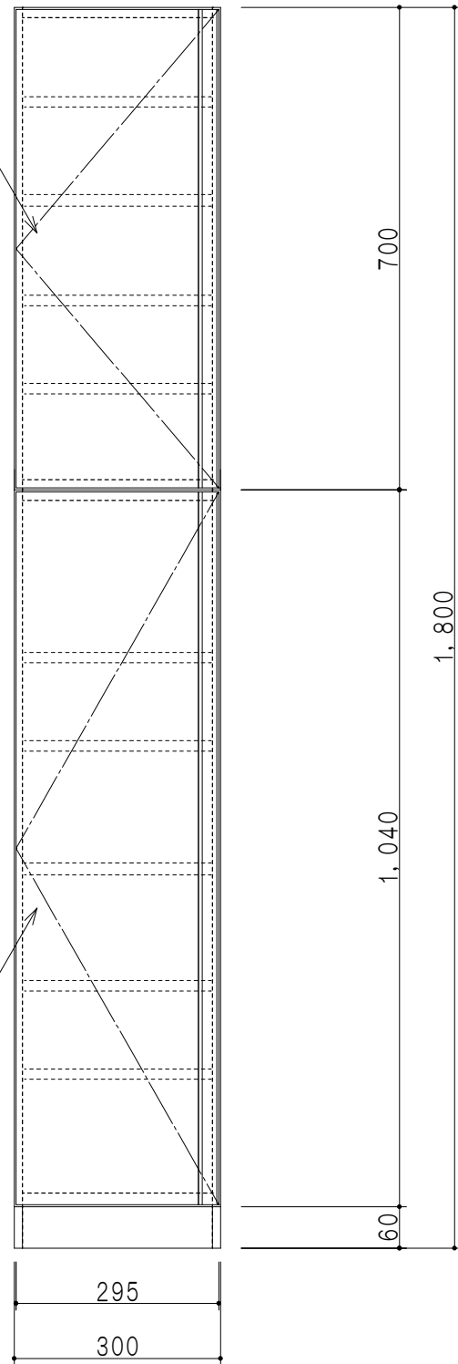
立面図
