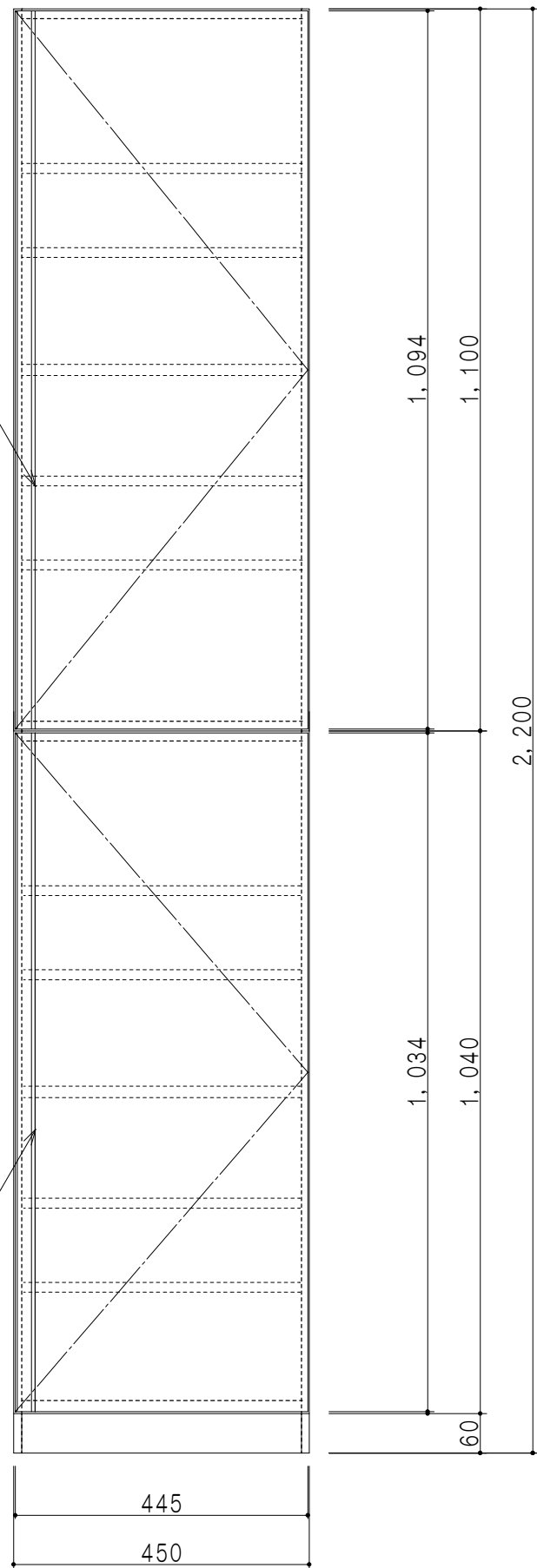
立面図
