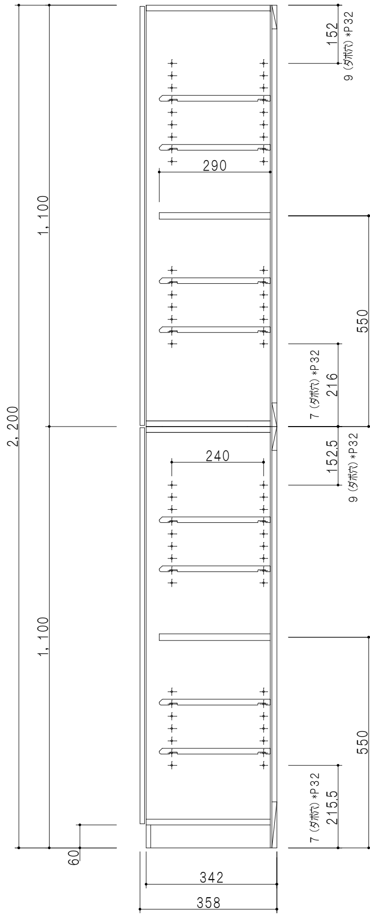
断面図
