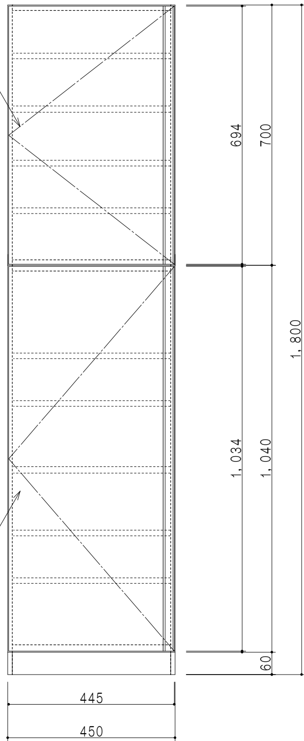
立面図
