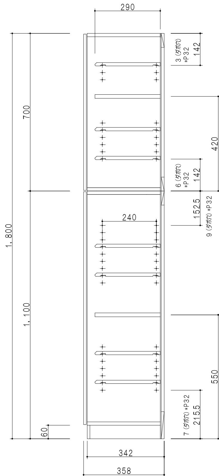
断面図
