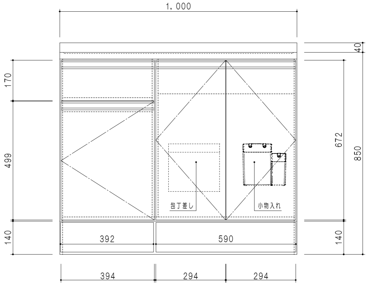
立面図
