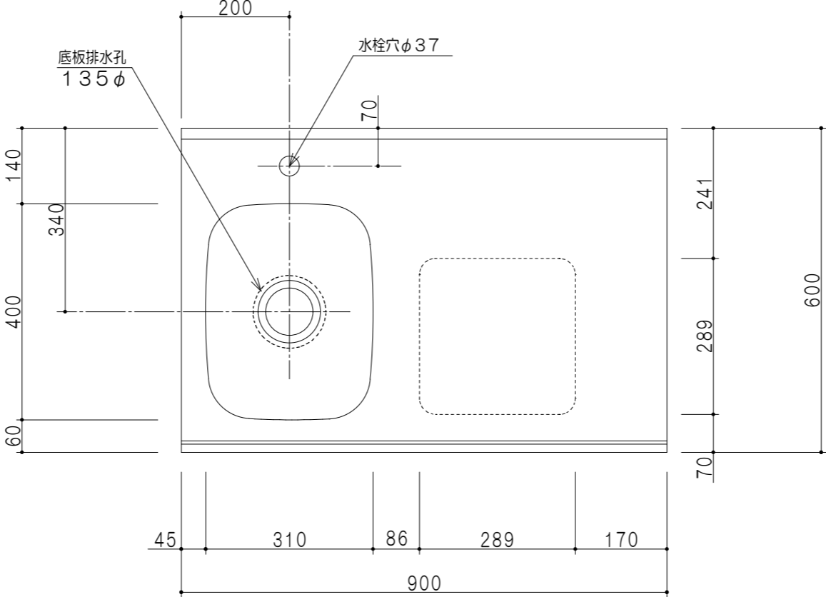
平面図
