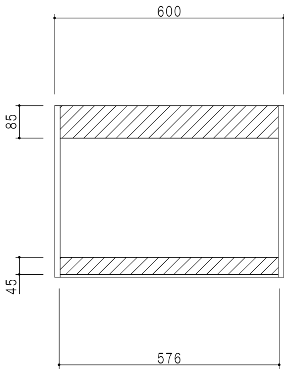
背面図
