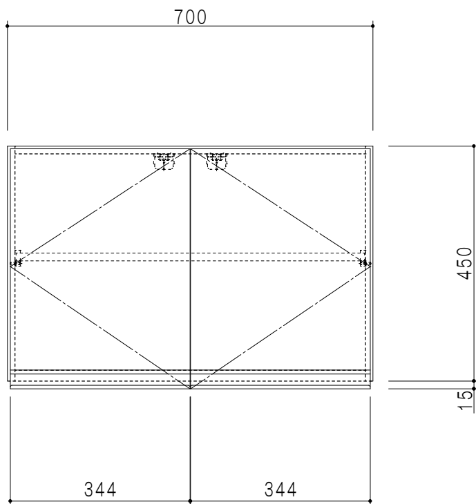
立面図
