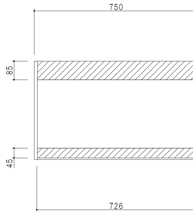
背面図
