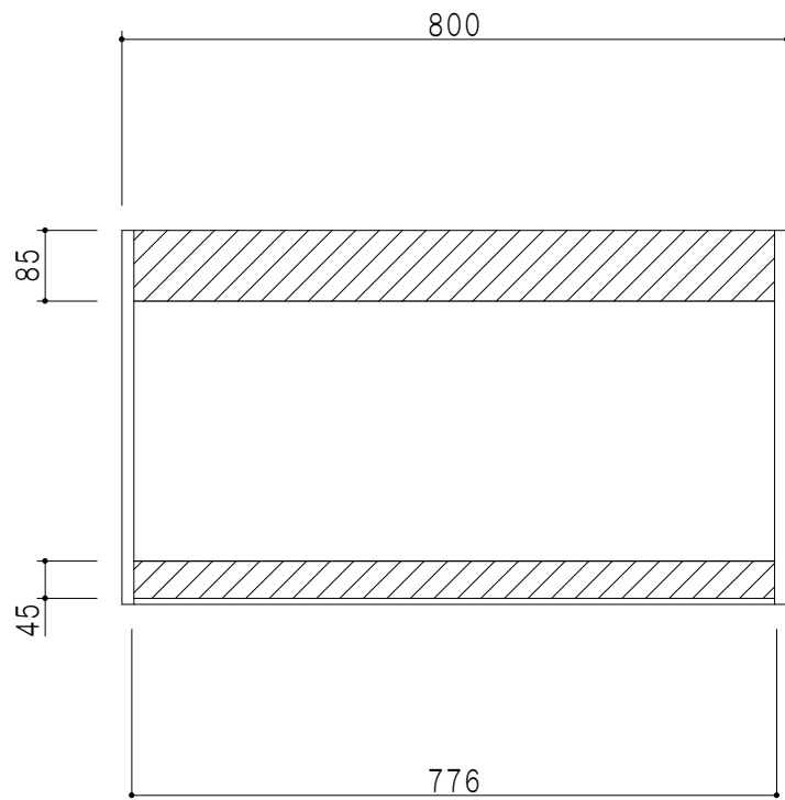
背面図
