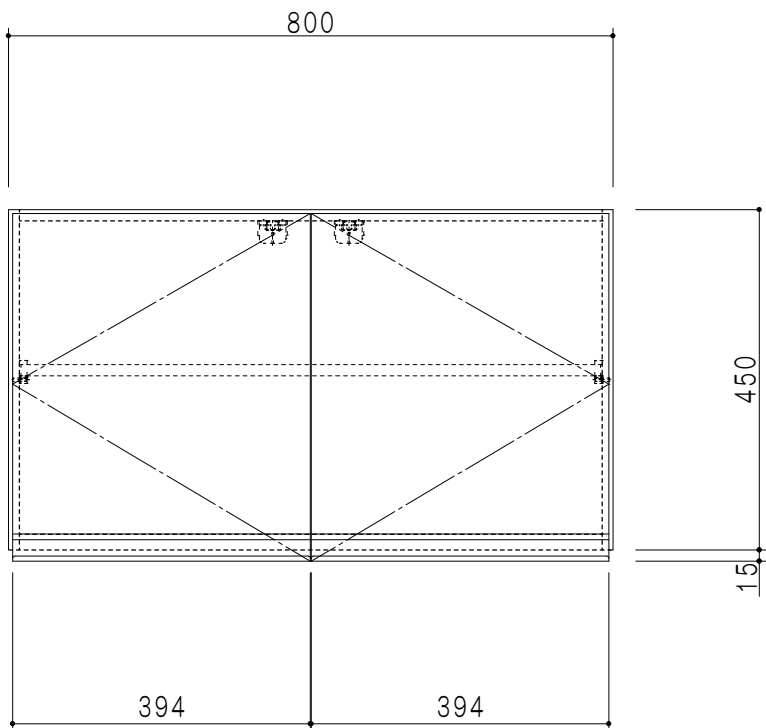
立面図
