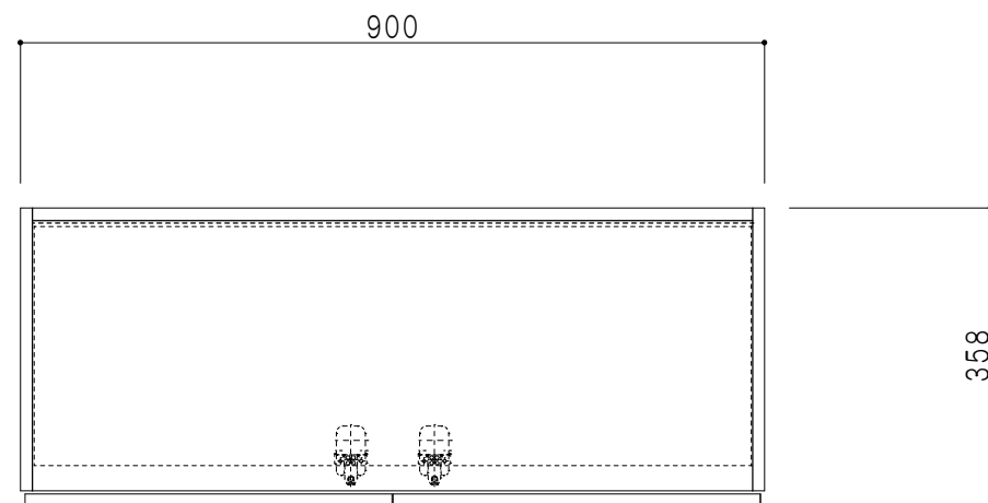
平面図
