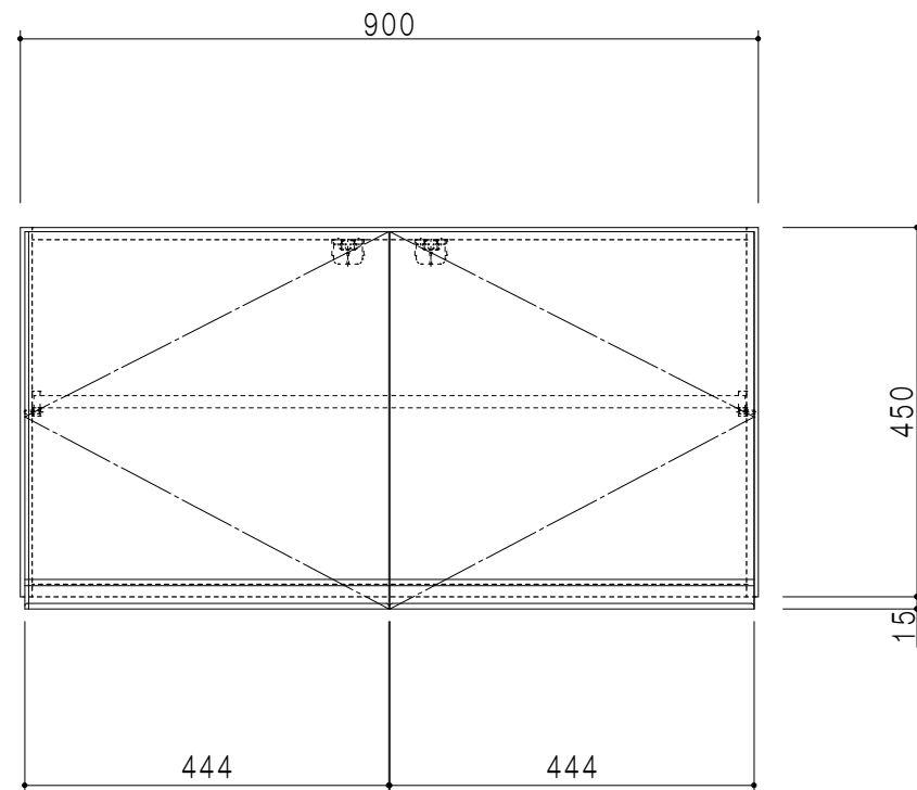
立面図
