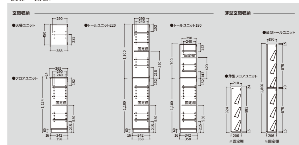
3点組み合わせタイプ SHO-80U + SHO-80TU + SHO-80F + SHO-80FT (34/38)
