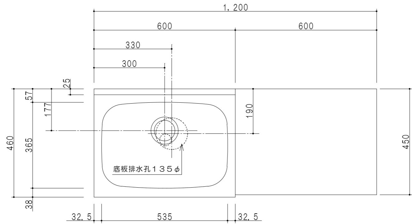
平面図
