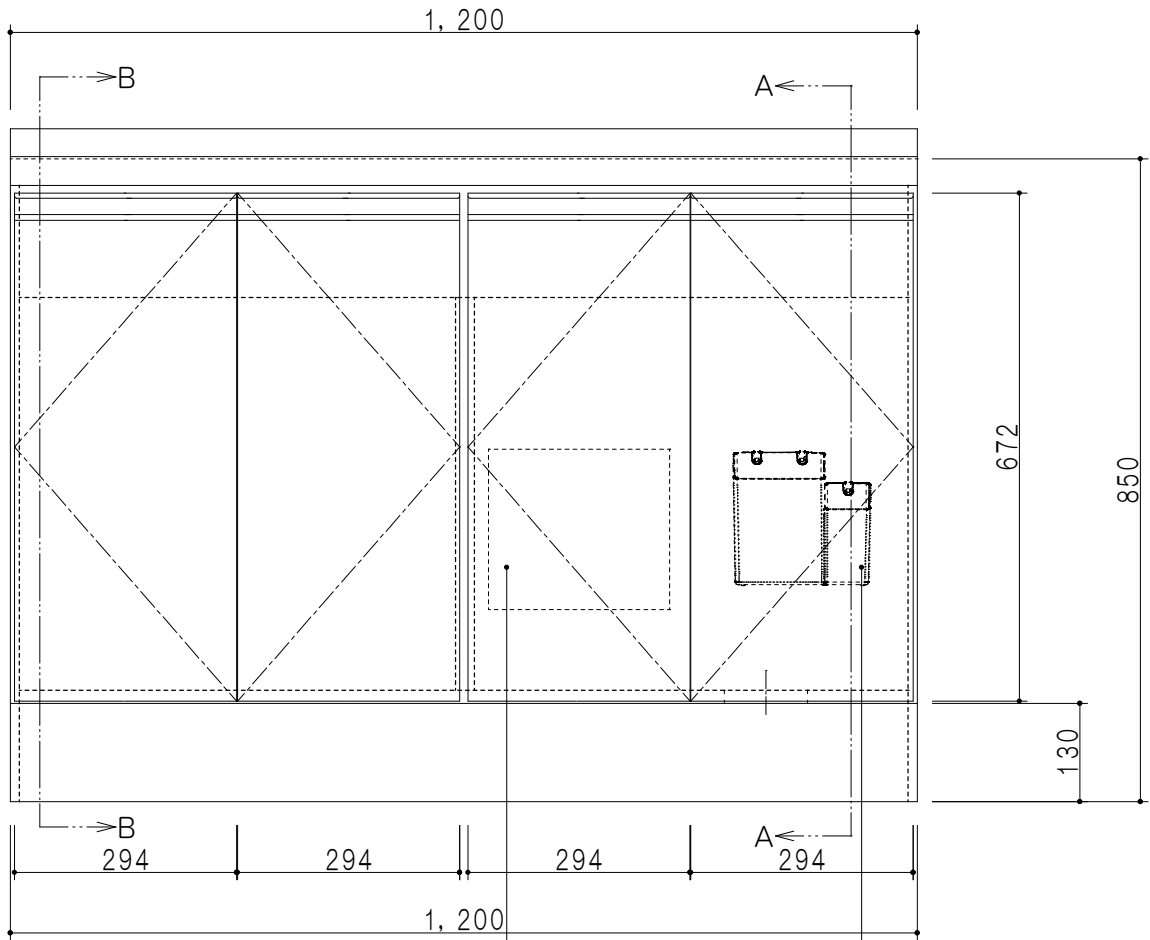
立面図
