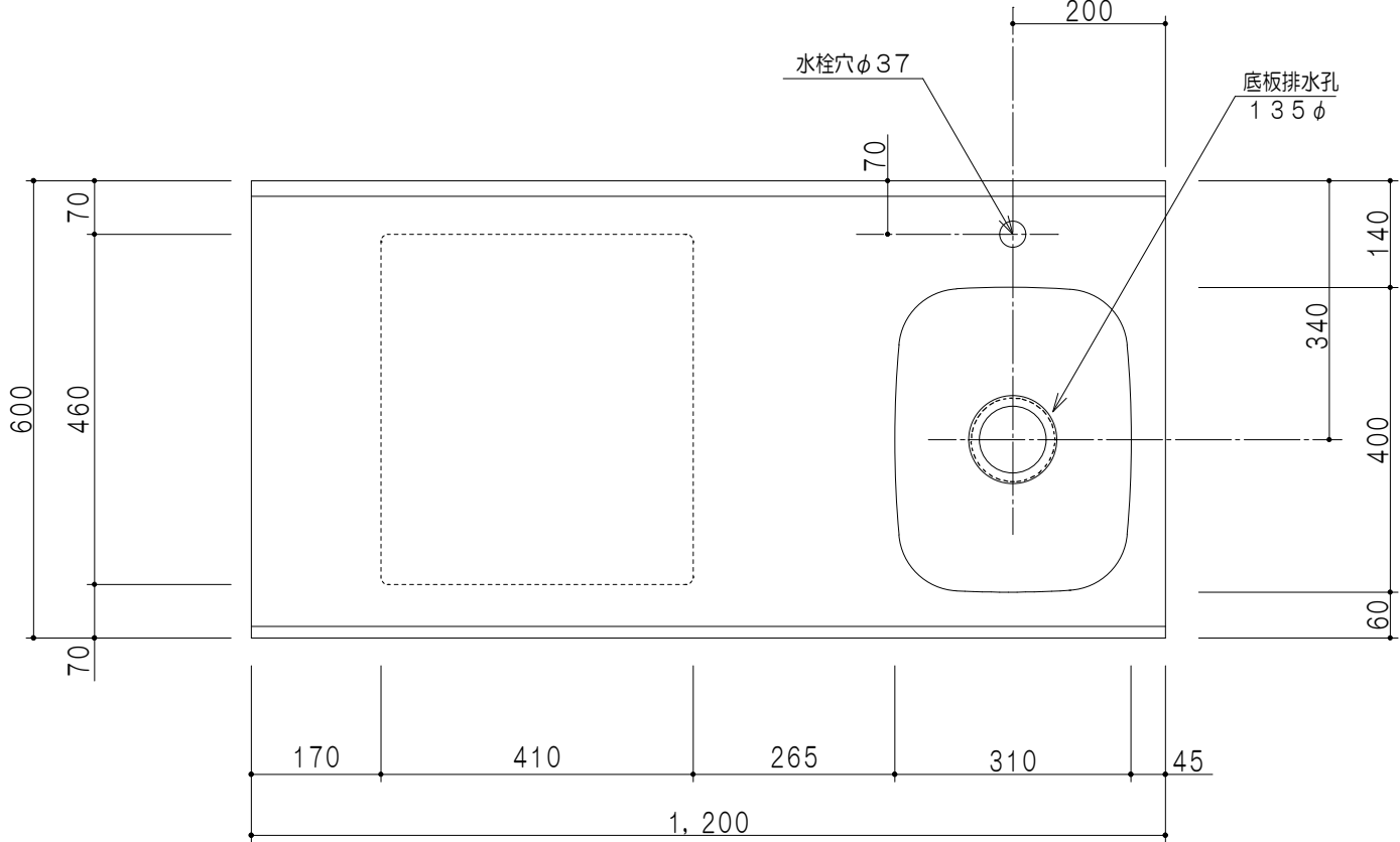
平面図
