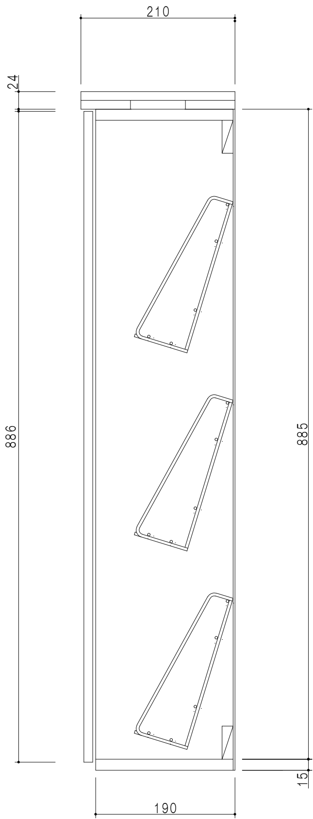
断面図
