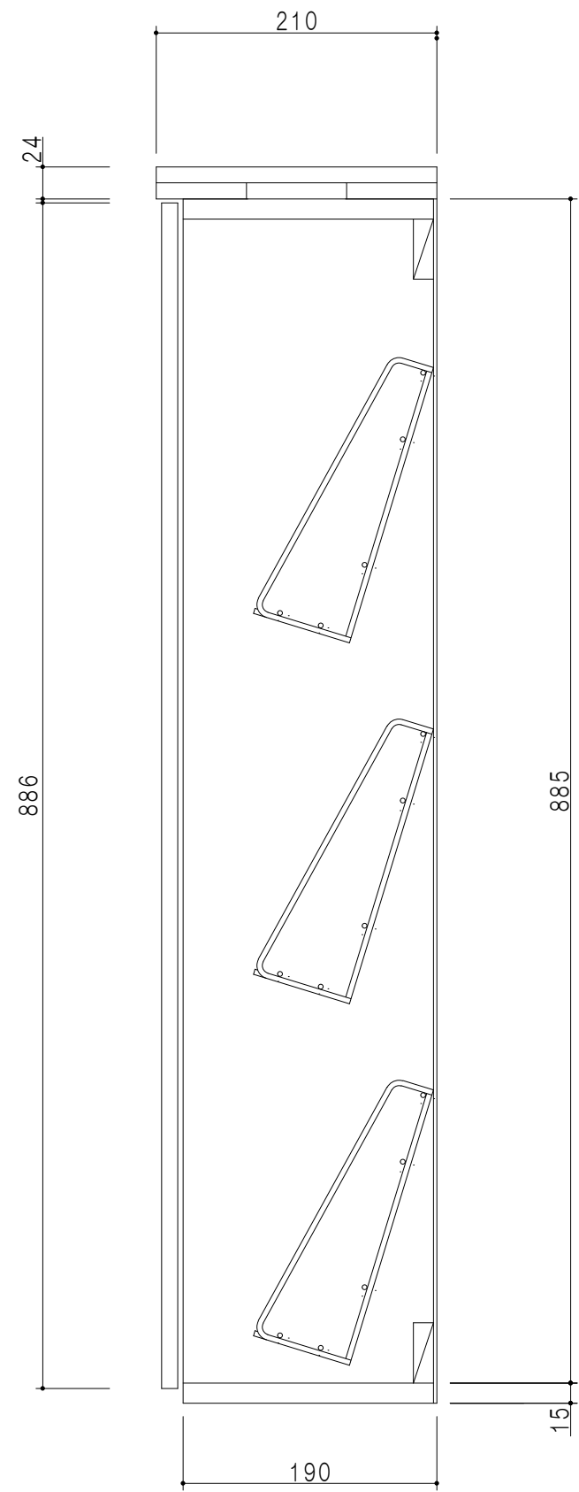
断面図
