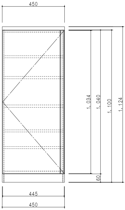
立面図
