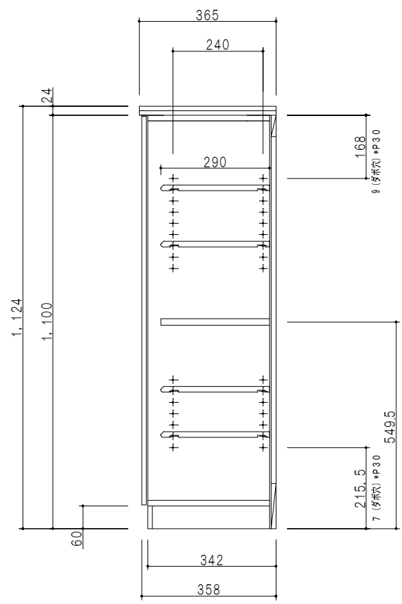
断面図
