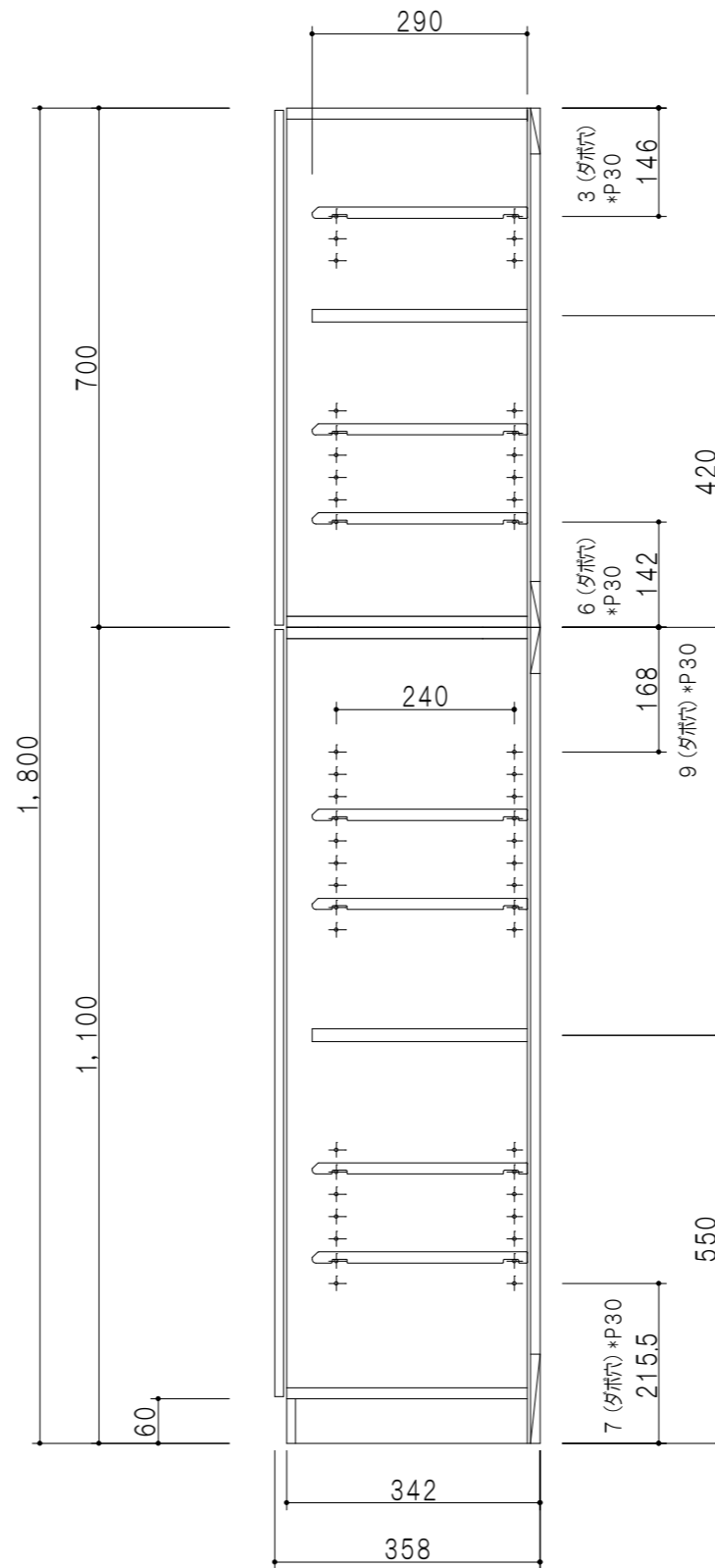
断面図
