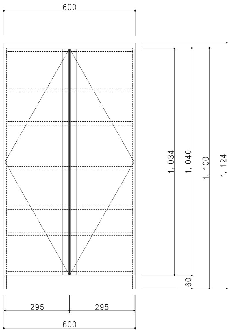
立面図
