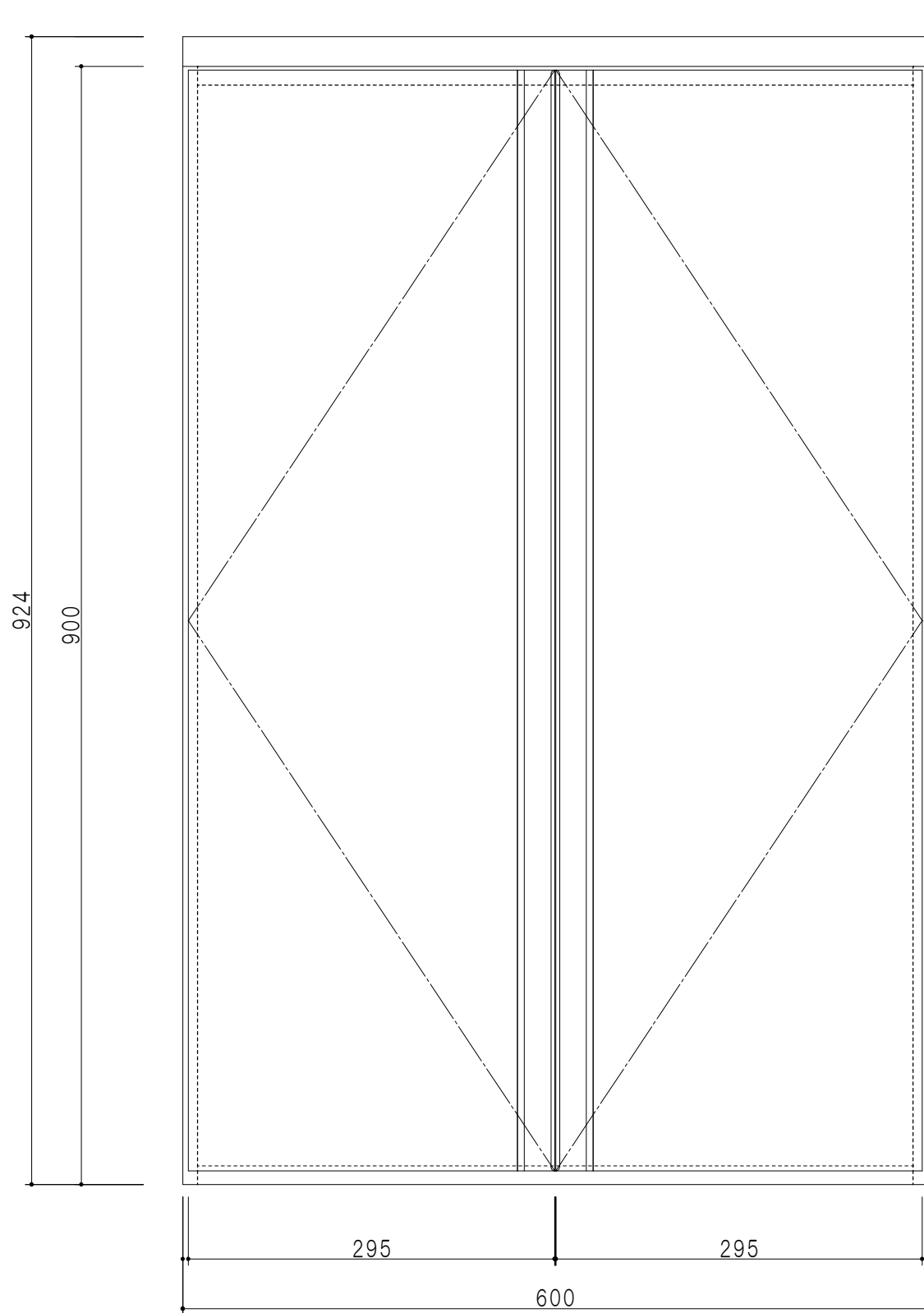
立面図
