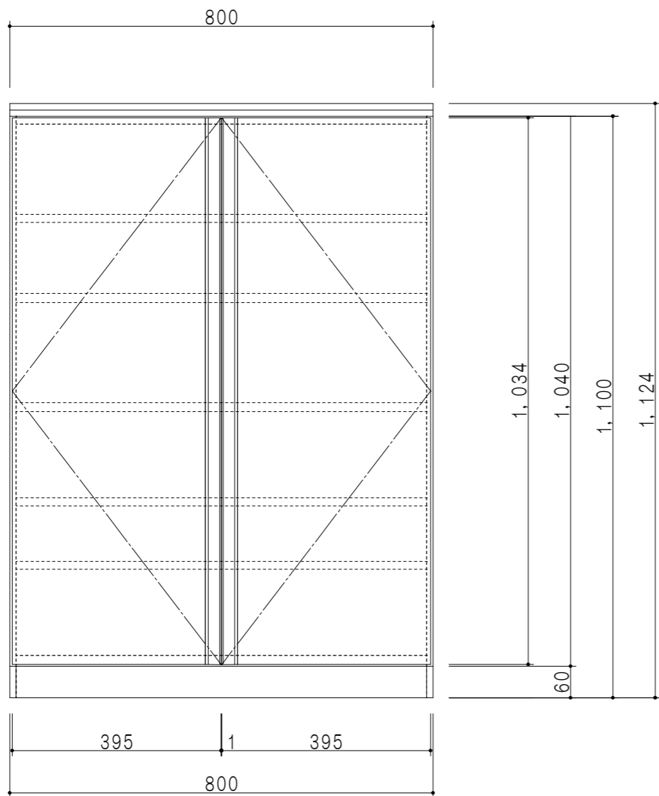
立面図
