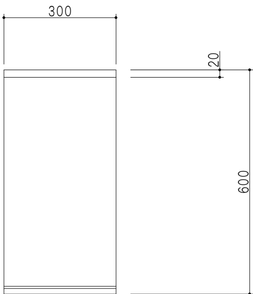
平面図
