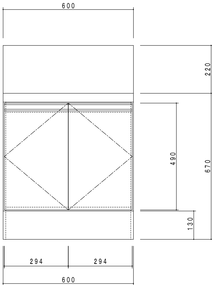
立面図
