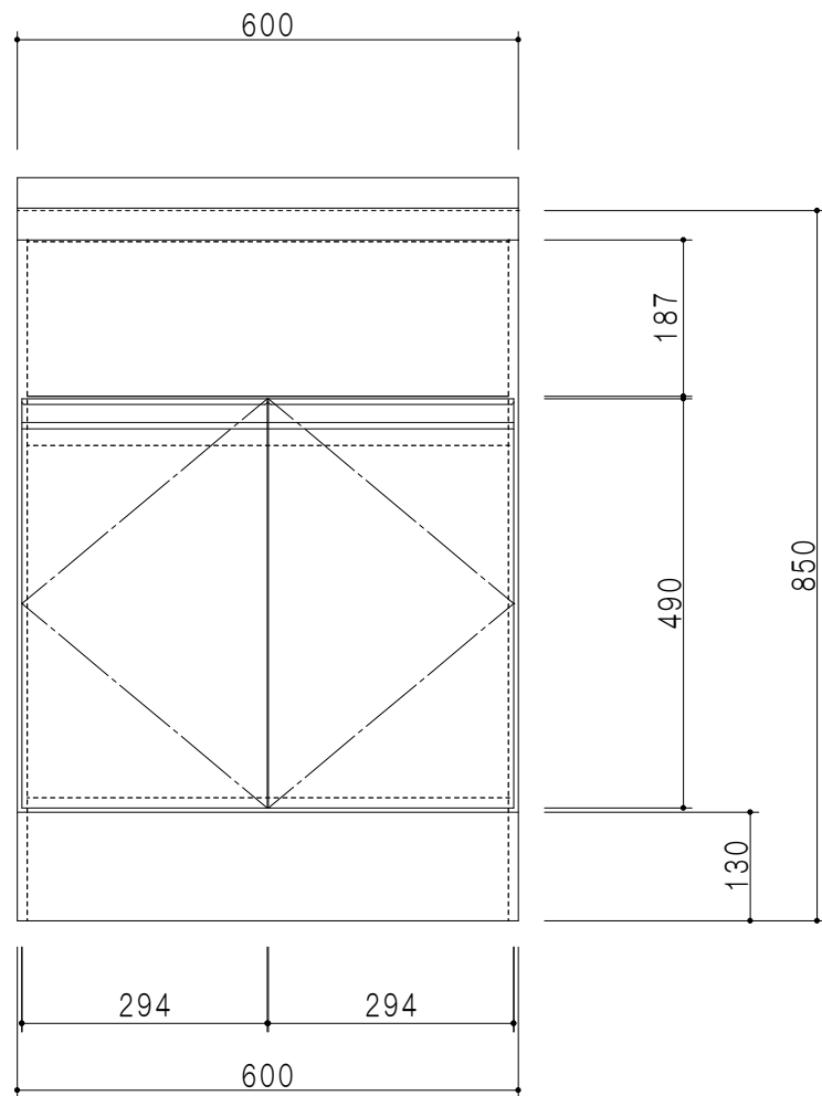
立面図
