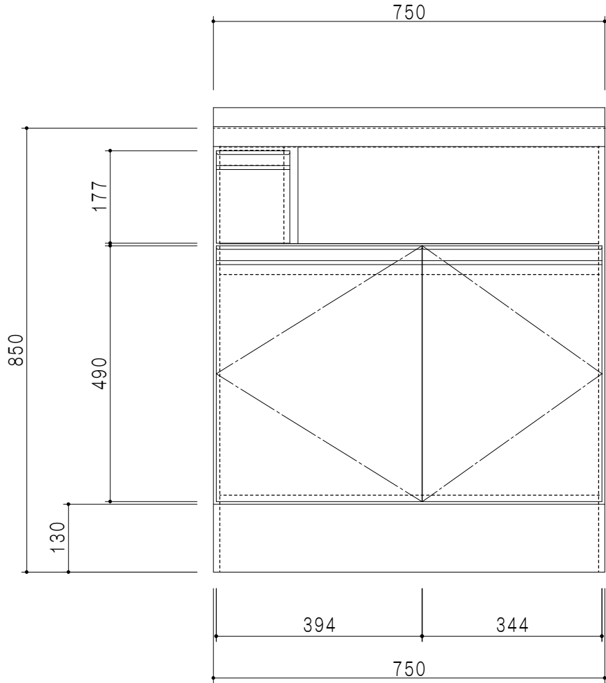
立面図
