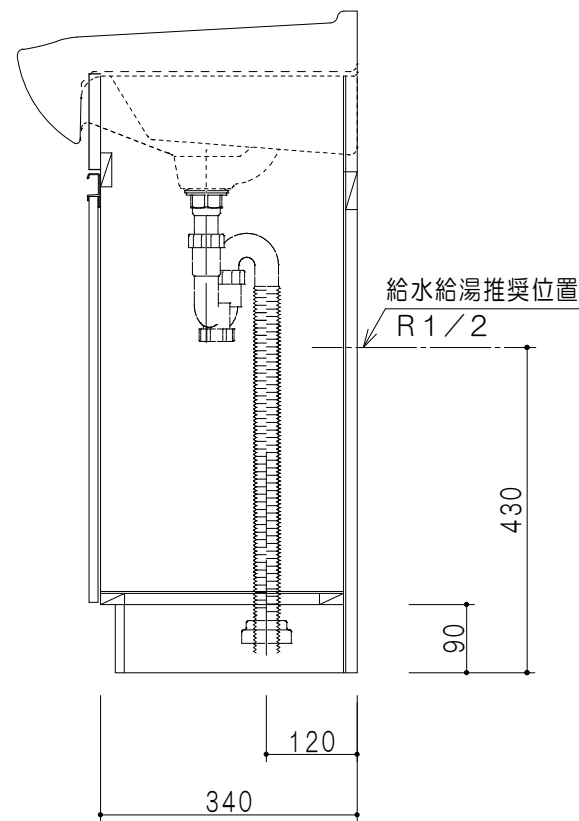
断面図
