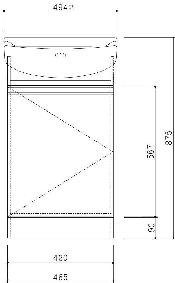
立面図
